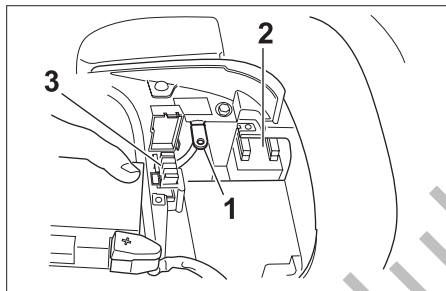
1. Отрицательный провод аккумуляторной батареи 2. Коробка главного предохранителя 3. Коробка плавких предохранителей
